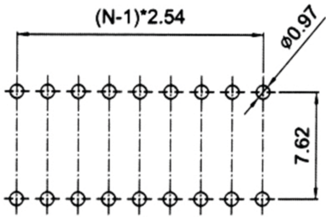
P.C.B LAYOUT
